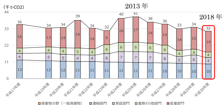
図2 部門・分野別の温室効果ガス（CO2）排出量の経年変化 図3 平成30年度部門・分野別構成比
